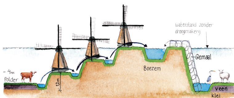
Principe des moulins en série en polderisation
